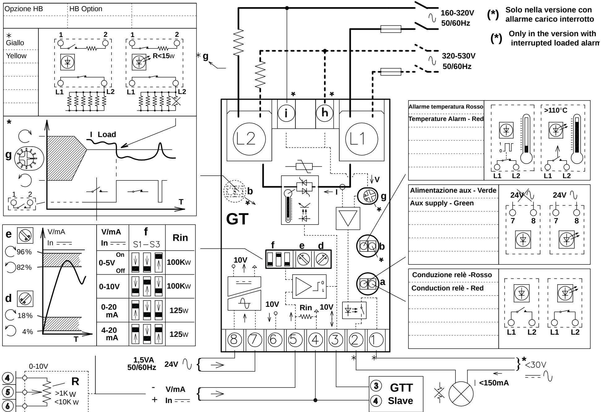
FIG. 1 Schéma de fonctionnement à blocs FIG. 1 Esquema funcional de bloques FIG. 1 Diagrama de bloco funcional
